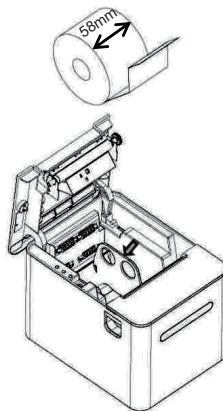
De installatielocatie van de 58mm papierrolgeleider is weergegeven in de afbeelding.
